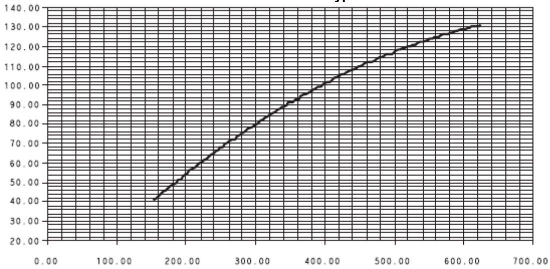
График заправки хладагента R123 при работе всех вентиляторов конденсатора Ось X -- Давление на клапане линии жидкости (PSIG) Ось Y -- Температура на клапане линии жидкости (°F)
